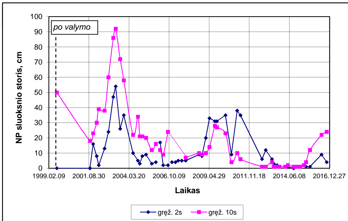
5 pav. Naftos produktų plėvelės storio dinamika buvusios Alytaus naftos bazės rajone
