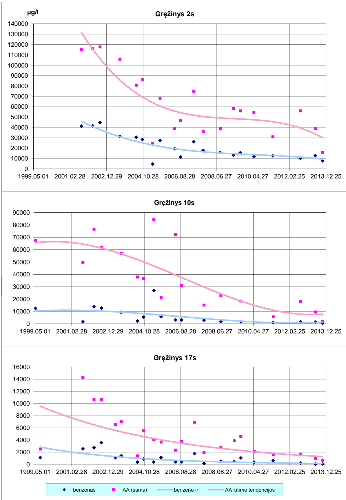
7 pav. Ištirpusių gruntiniame vandenyje aromatinių angliavandenilių (AA) ir benzeno koncentracijų kitimas gręžiniuose 2s, 10s ir 17s
