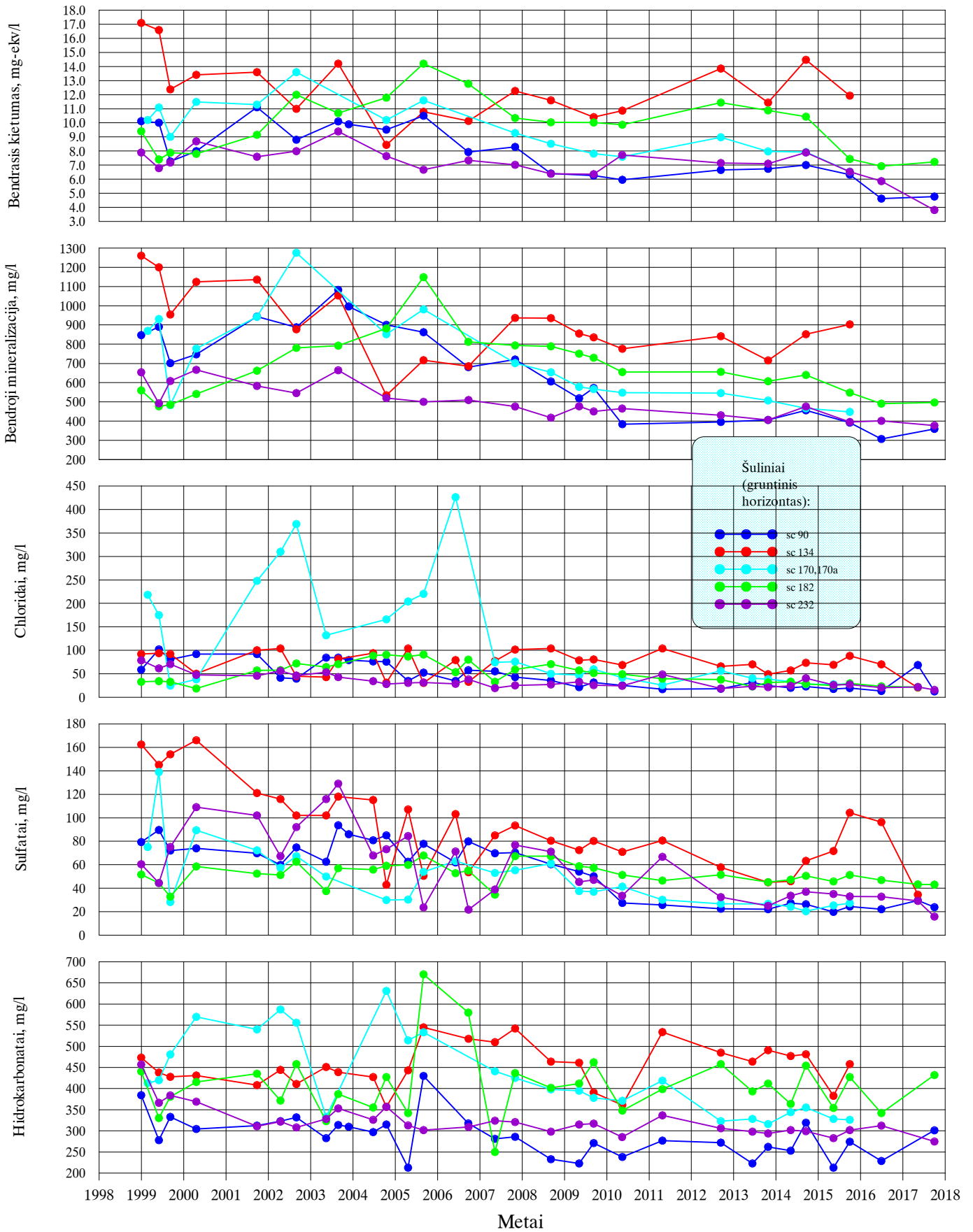
6 pav. Kai kurių rodiklių verčių kitimas gruntiniame vandenyje monitoringo taškuose sc90 (sc90a), sc134, sc170 (sc170a), sc182, sc232
