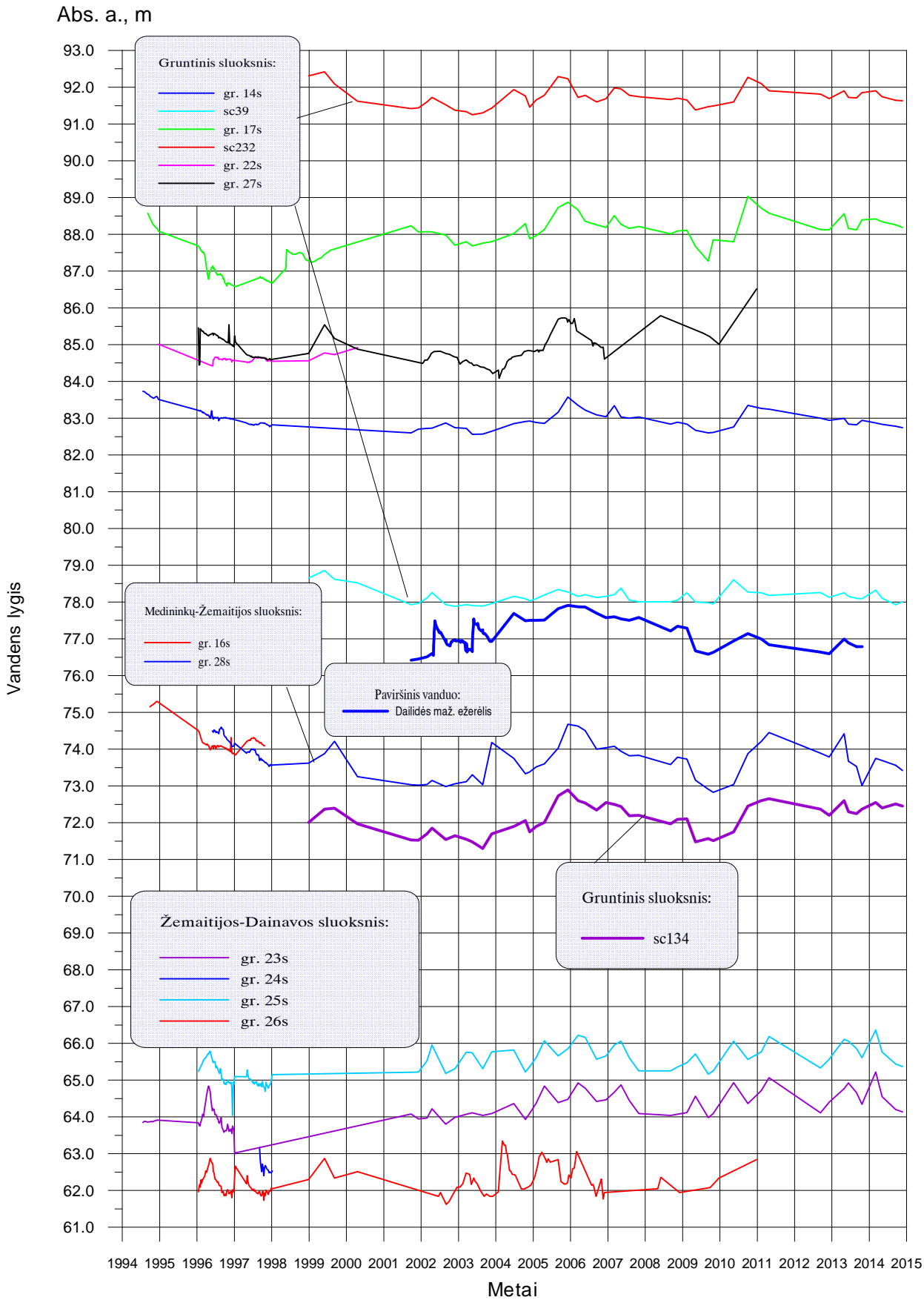
3 pav. Požeminio vandens lygio Alytuje svyravimų grafikai
