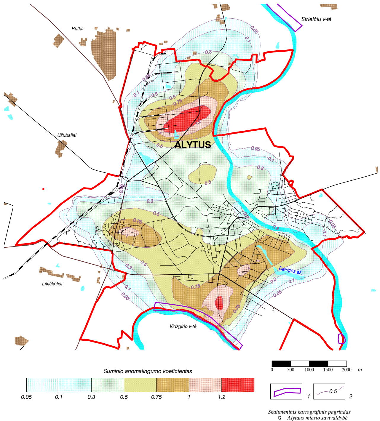
4.5 pav. Prognozinis 2000 m. buvusių gruntinio horizonto užterštumo anomalijų poveikis Žemaitijos-Dainavos vandeningajam horizontui, ateityje 25 metus eksploatuojant Strielčių ir Radžiūnų vandenvietes debitu, atitinkančiu patvirtintų išteklių kiekį, o Vidzgirio vandenvietės neeksploatuojant
